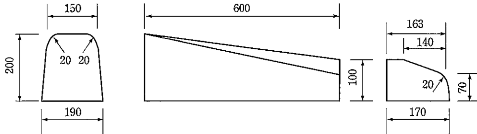
両面A切下 M2
